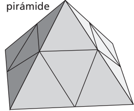
pirámide
