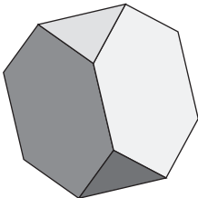
tetraedro truncado
