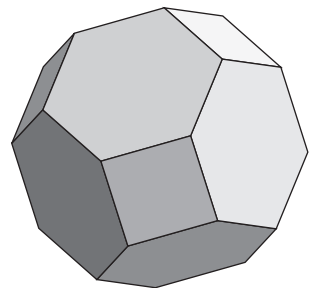
octaedro truncado
