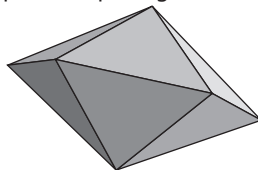
bipirámide pentagonal
