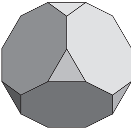
cubo truncado
